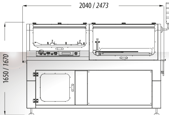
LA-6000CS / LA-8000CS4 (mm)
